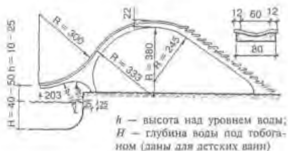
Тобоган железобетонный Разрез по желобу
